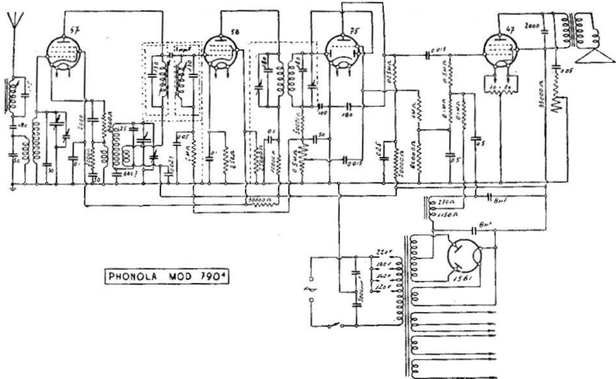
PHONOLA-RADIO (S. A. FIMI). — Modelli: « 790 1 e .791 1 ». - Produzione 1935. - Media frequenza: 470 kHz
