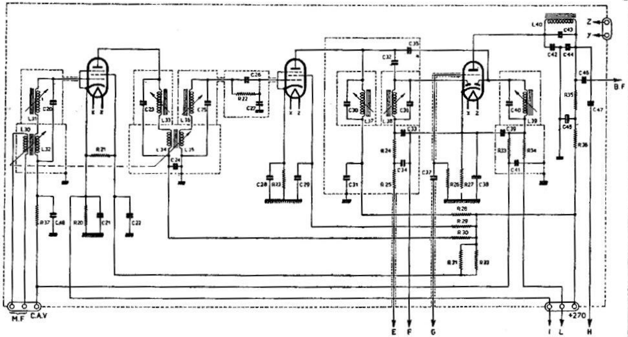
Schema elettrico A. F. Vedi tavola R. 8279 (5/11)
