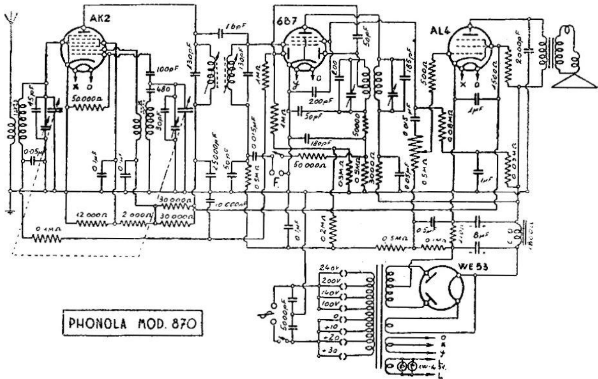
PHONOLA (S. A. FIMI). — Modelli « 870, 871 e 873 ». - Produzione 1937. - Media freq.: 470 k Hz.
