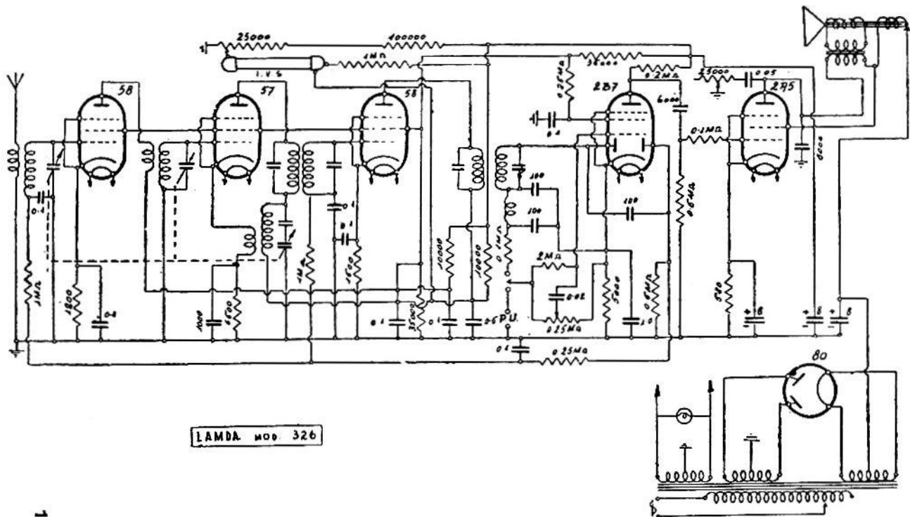
OLIVIERI e GLISENTI. — Modello « Lamda 326 ». - Produzione 1933 ». - Media frequenza: 175 kc.
