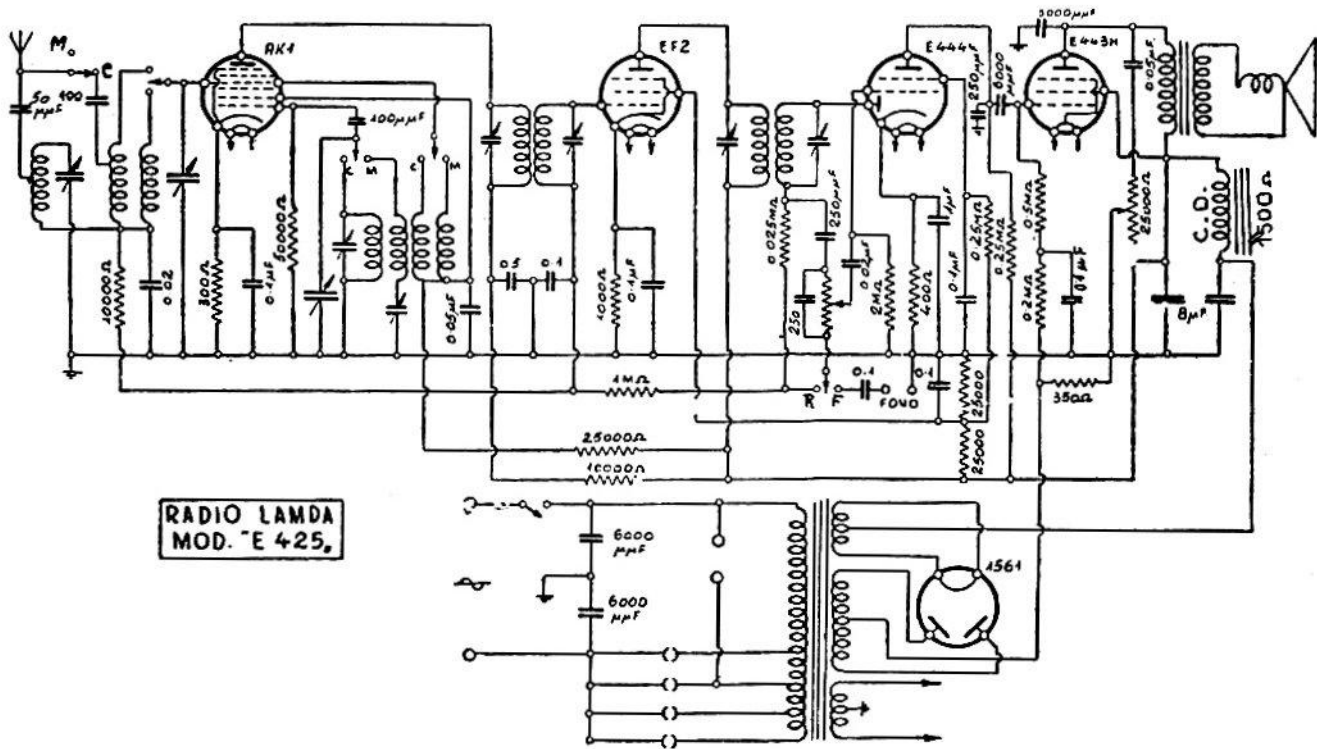
OLIVIERI E GLISENTI. — Modello « Lamda F.425 ». • Produzione 1934. • Media frequenza: 175 kc.
