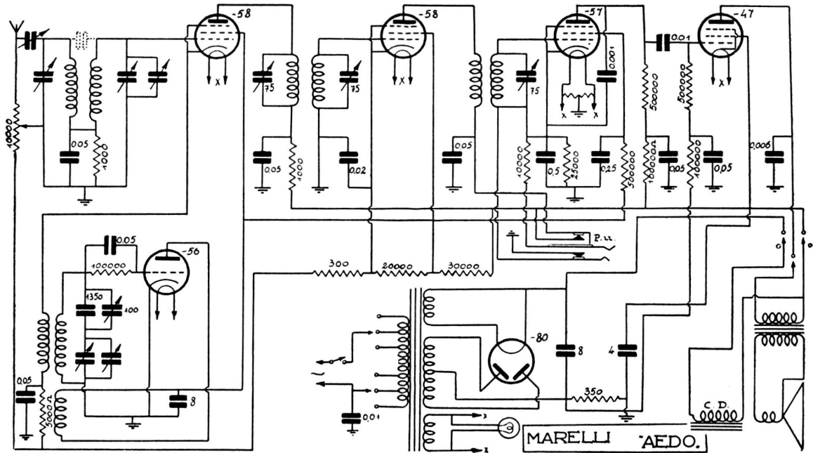
Onde medie. - M. F. 485 kc. - Oscillatrice 56 separata.
