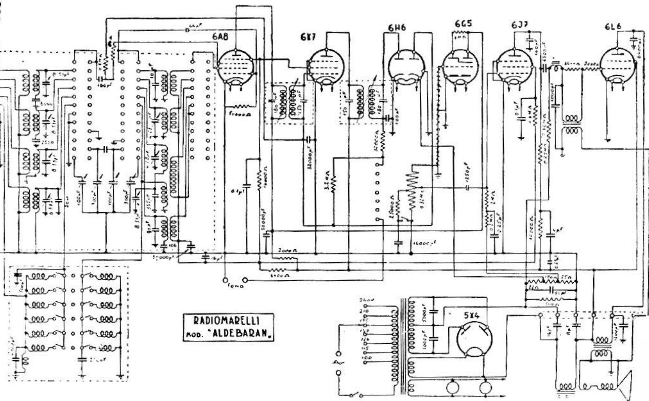
RADIO MARELLI. — Modelli Aldebaran e Aldebaran fono. — Produzione 1938-39. — Gamme: cc. (19-30), c. (30-50), m. (200-570), l. (1000-2000). — Potenza d'uscita 5,5 W. — Media frequenza: 450 kHz.
