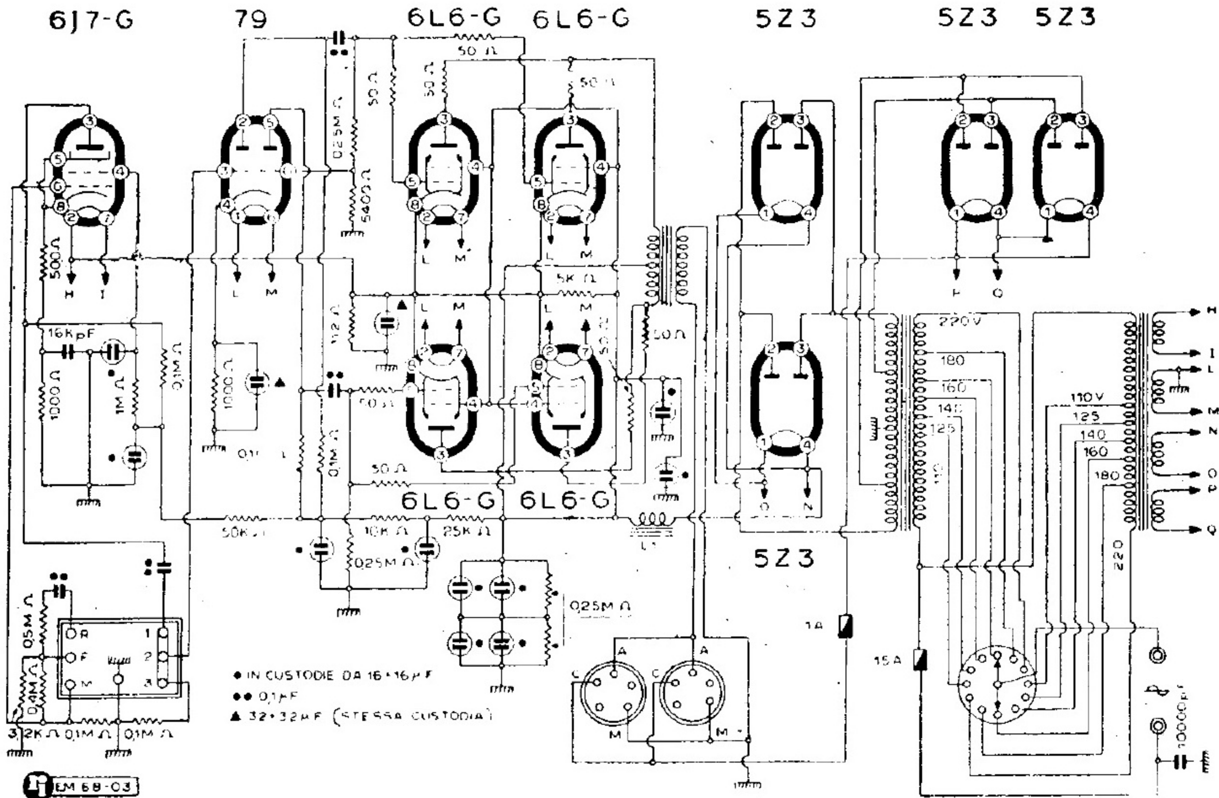
MAGNETI MARELLI - AMPLIFICATORE MOD. « AP 22 »
