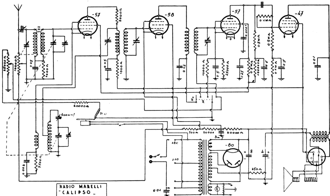
Onde medie. - M. F. 465 kc. - Preselettore. - 57 oscill.-modul.; 58 amplif. m. f.; 57 demodul.; 47 finale a polarizzazione fissa. - Potenza d'uscita: 2,5 watt.
