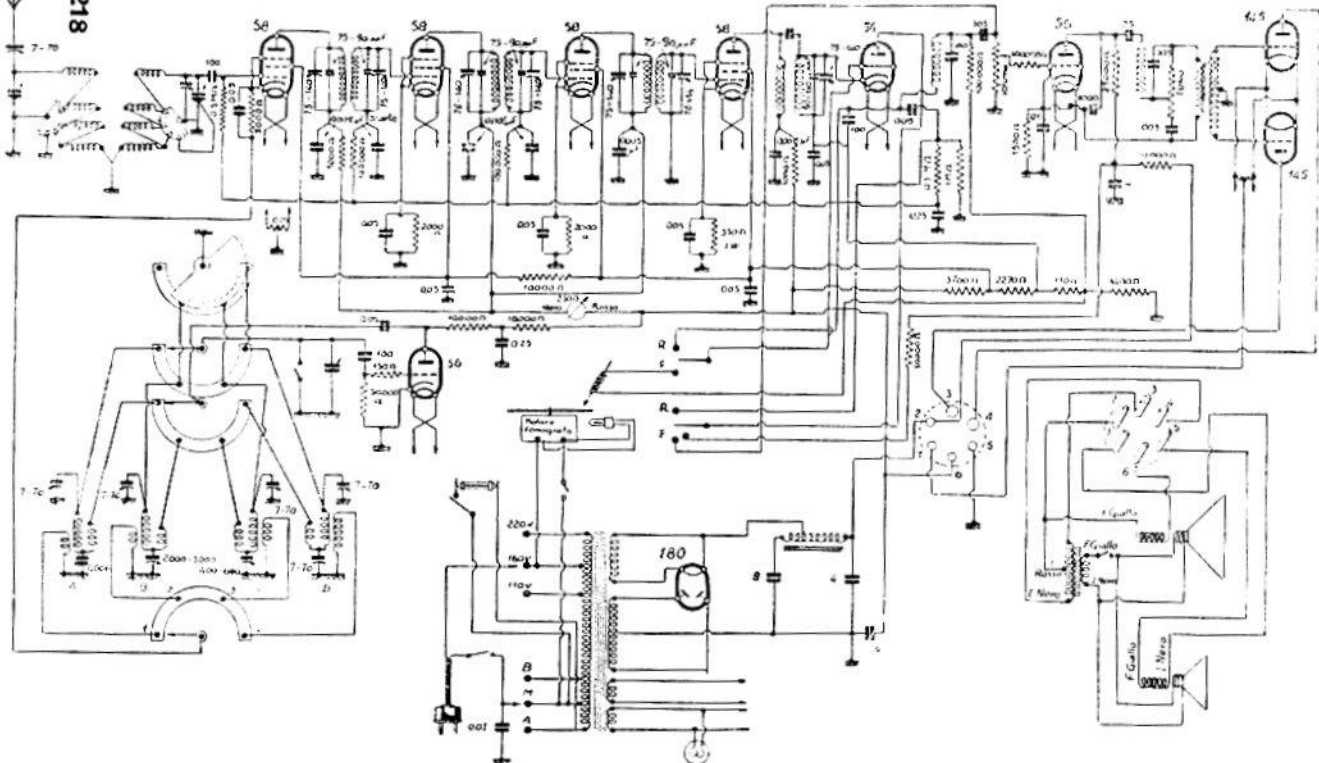
RADIO MARELLI. — Mod. « Argeste » e « Fonoargeste ». — MF: 125 kHz. — Produzione 1934-35.
