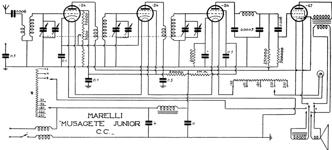
Onde medie. - Amplificazione diretta in alta frequenza con due valvole 24, seguita da una demodulatrice pure 24 e dalla finale 47. - Alimentazione con corrente continua della rete. - Potenza d'uscita: 2 watt.
