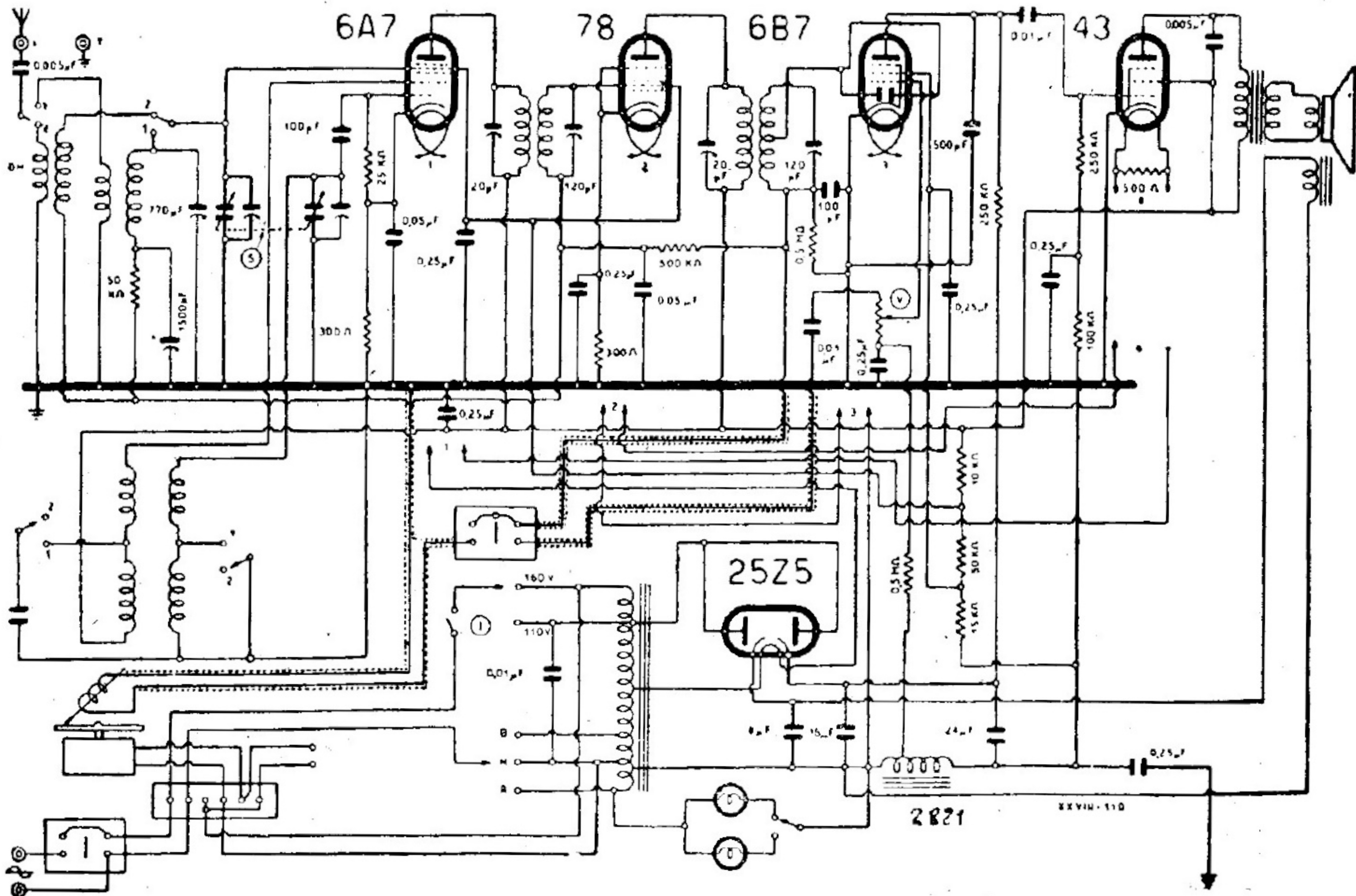
RADIOMARELLI . MOD. « VERTUMNO II »
