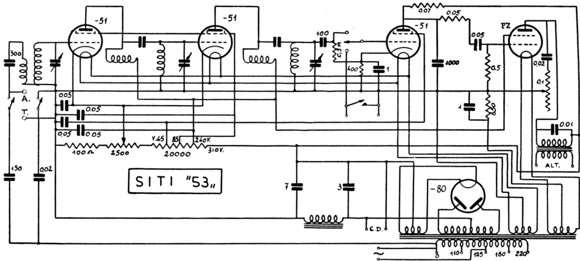
Onde medie. - Amplificazione diretta in a. f. con due schermate 51. - Demodulatrice 51. - Finale PZ (47). - Potenza d'uscita: 2,5 watt.
