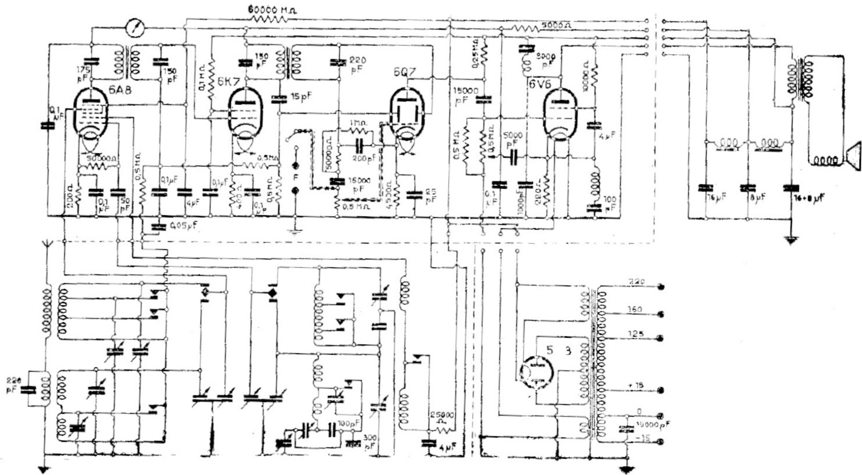
RADIO SUPERLA - MODD. « 550 » « 1550 »
