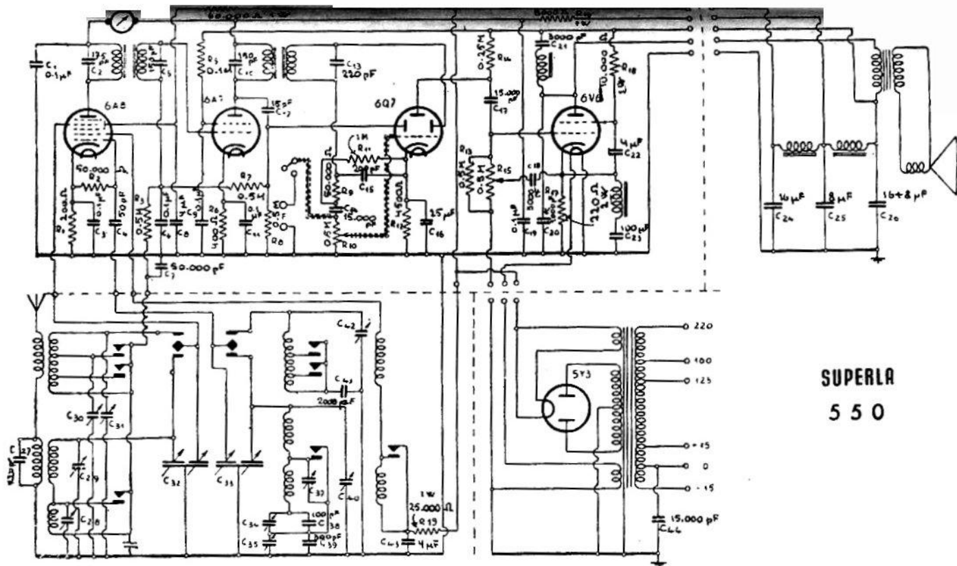
RADIO SUPERLA. — Mod. « 550 » e « 1550 » (prima e seconda serie). — Produzione 1939-1940. — Media frequenza: 468 kHz. — 5 gamme d'onda. — Gamme d'onda: C1 (12,1-20,5 m.), C2 (18,7-32 m.), C3 (30-51,2 m.), m. (200-600), l. (700-2000 m.). — (Le Note di Servizio si trovano in Servizio Radiotecnico, vol. II).
