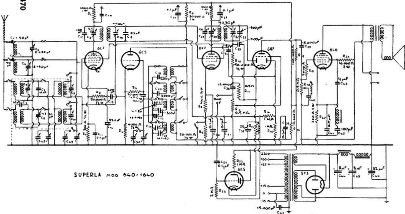
RADIO SUPERLA. — Mod. « 640 » e « 1640 ». — Produzione: 1939-1940. — Media frequenza: 4 \frac{1}{2} kHz. — Gamme: c. c. (13,5-25 m), c. (19-50 m), m. (200-600 m), l. (700-2000 m). — Potenza d'uscita: ca. 1 watt.
