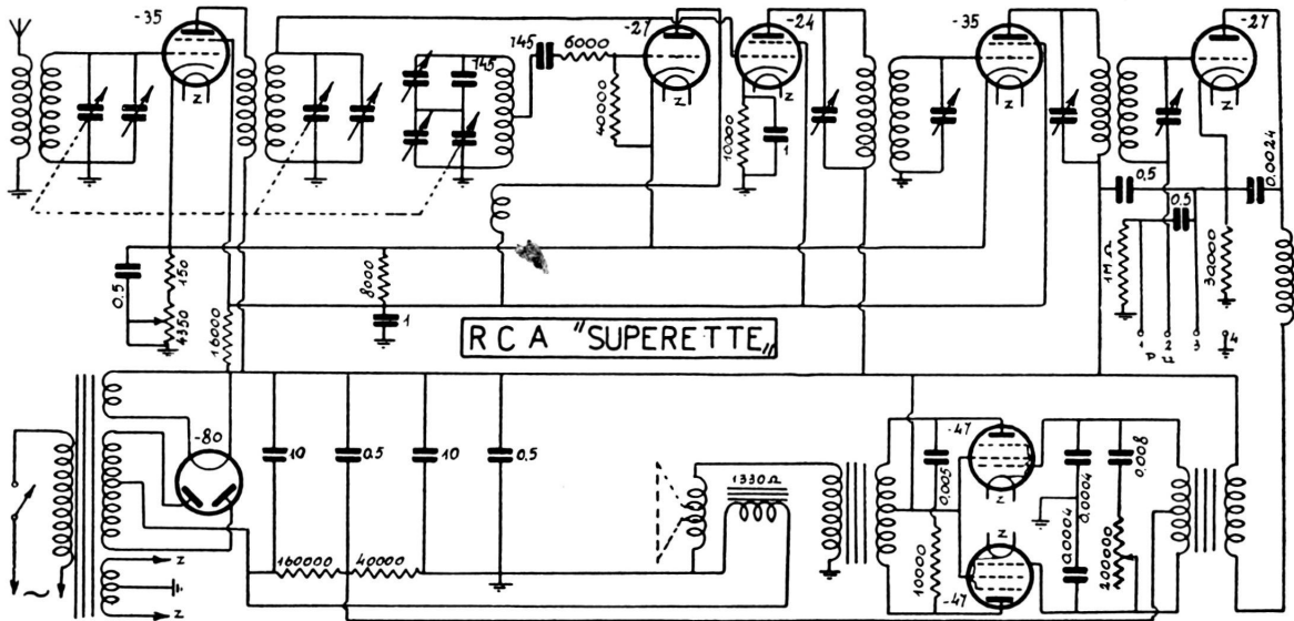
Onde medie. - M. F. 175 kc. - 35 amplif. in a. f. - 27 oscillatrice separata. - 24 modulatrice. - 35 amplif. m. f. - 27 demodulatrice. - Controfase di 47 finali. - Potenza d'uscita: 4,5 watt.
