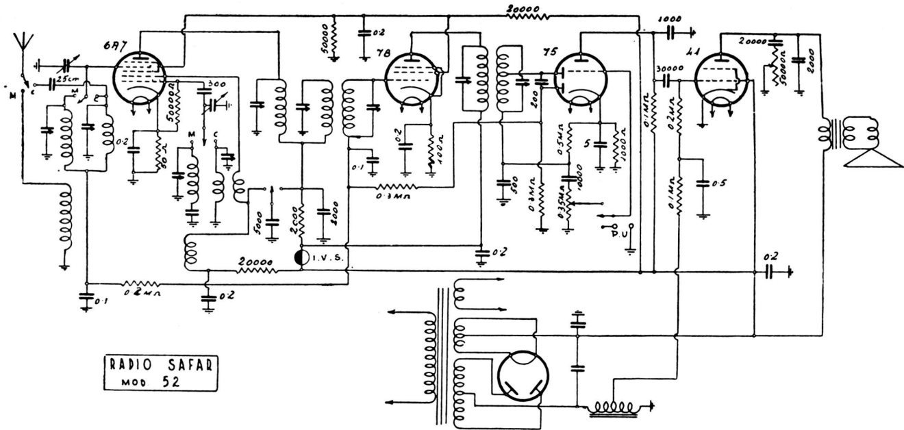
Onde medie e corte. - M. F. 175 kc. - C. A. V. - C. T. - Indicatore ottico di sintonia. - Scala parlante. - Lo stesso chassis anche nel radiofonografo mod. 52 RF. - Potenza d'uscita: 3 watt.
