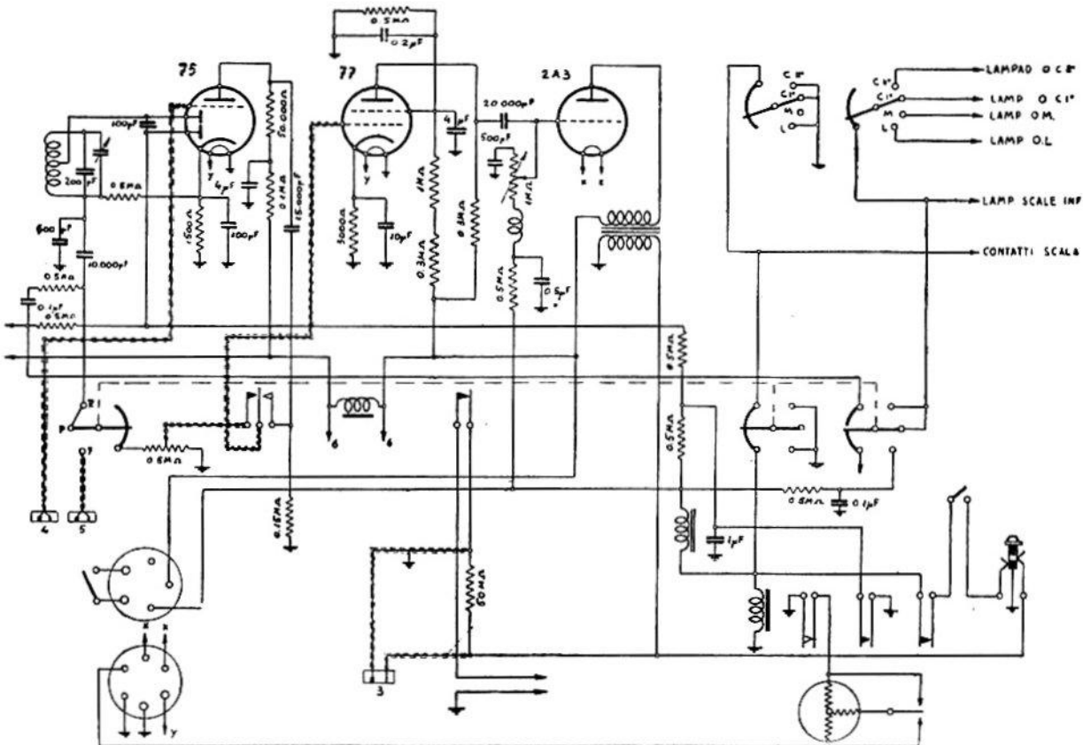
RADIO SAFAR. — Mod. « 844 ». — Parte rivelatrice e finale. (Per la parte AF e MF v. schema precedente).
