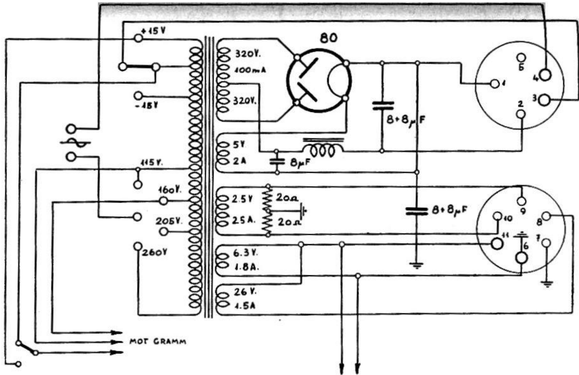
RADIO SAFAR. — Mod. « 844 ». — Parte alimentatrice. (Per le parti amplificatrice e rivelatrice v. schemi 832 e e 833).
