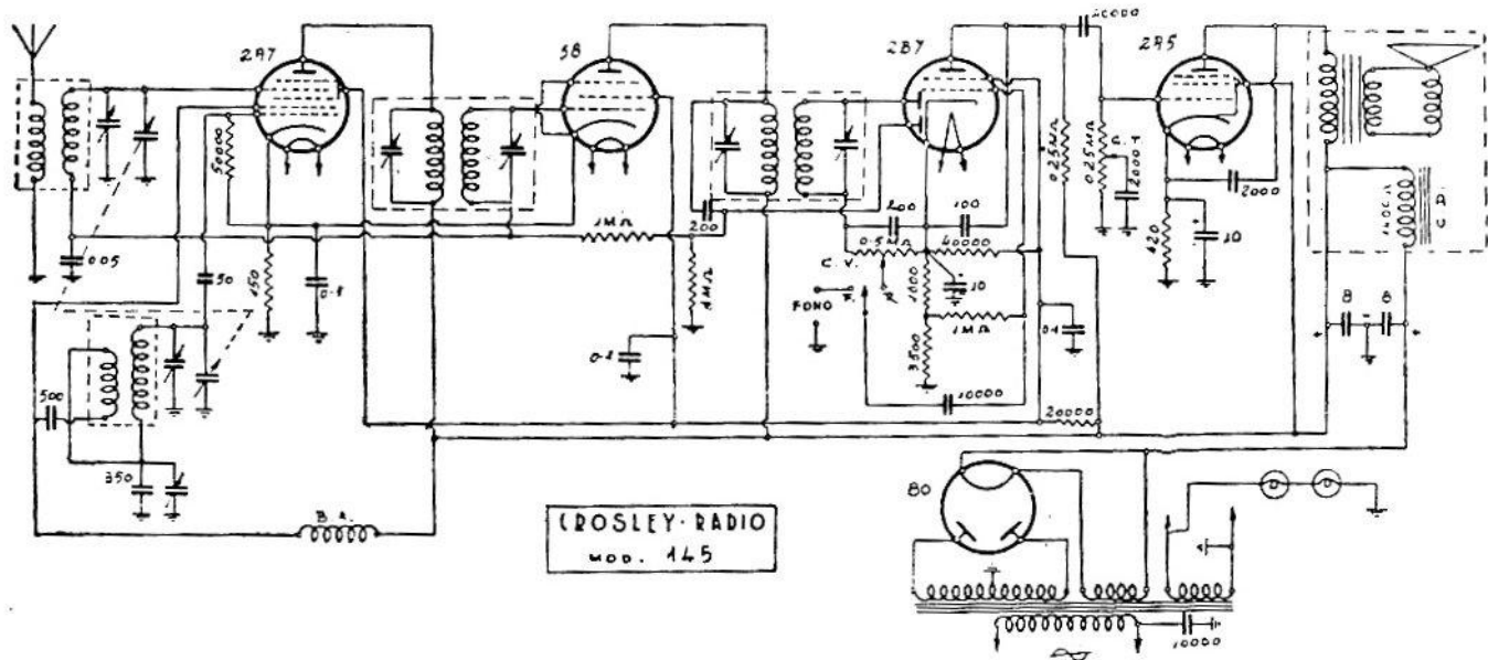
CROSLEY RADIO — Modello «145», - Produzione 1934. - Media frequenza: 350 kc.
