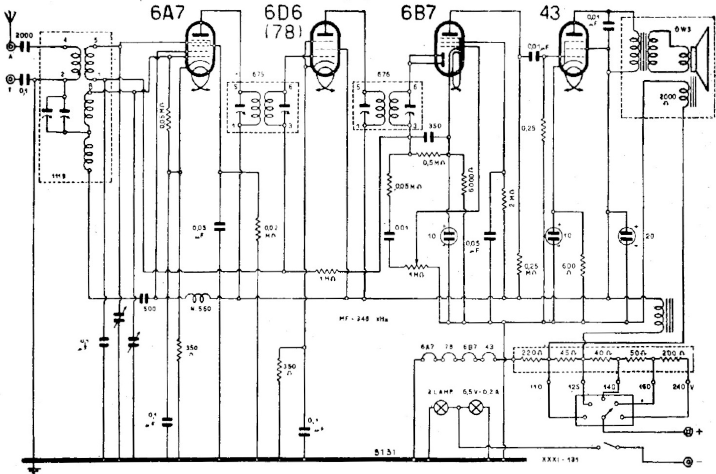
S.I.A.R.E. CROSLEY - MOD. « 7411 D. C. »
