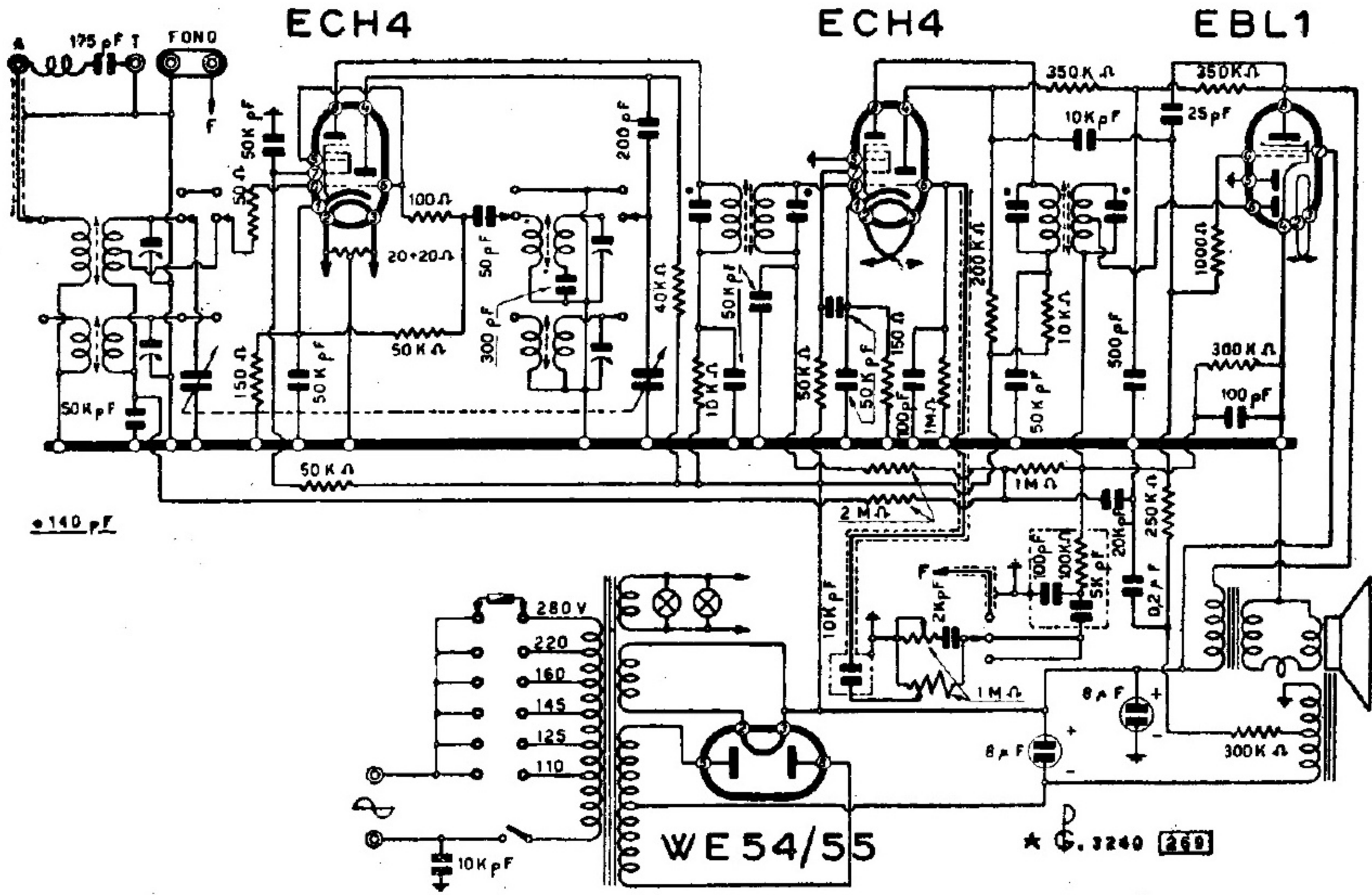
SIEMENS S. A. - MOD. « S 425 »
