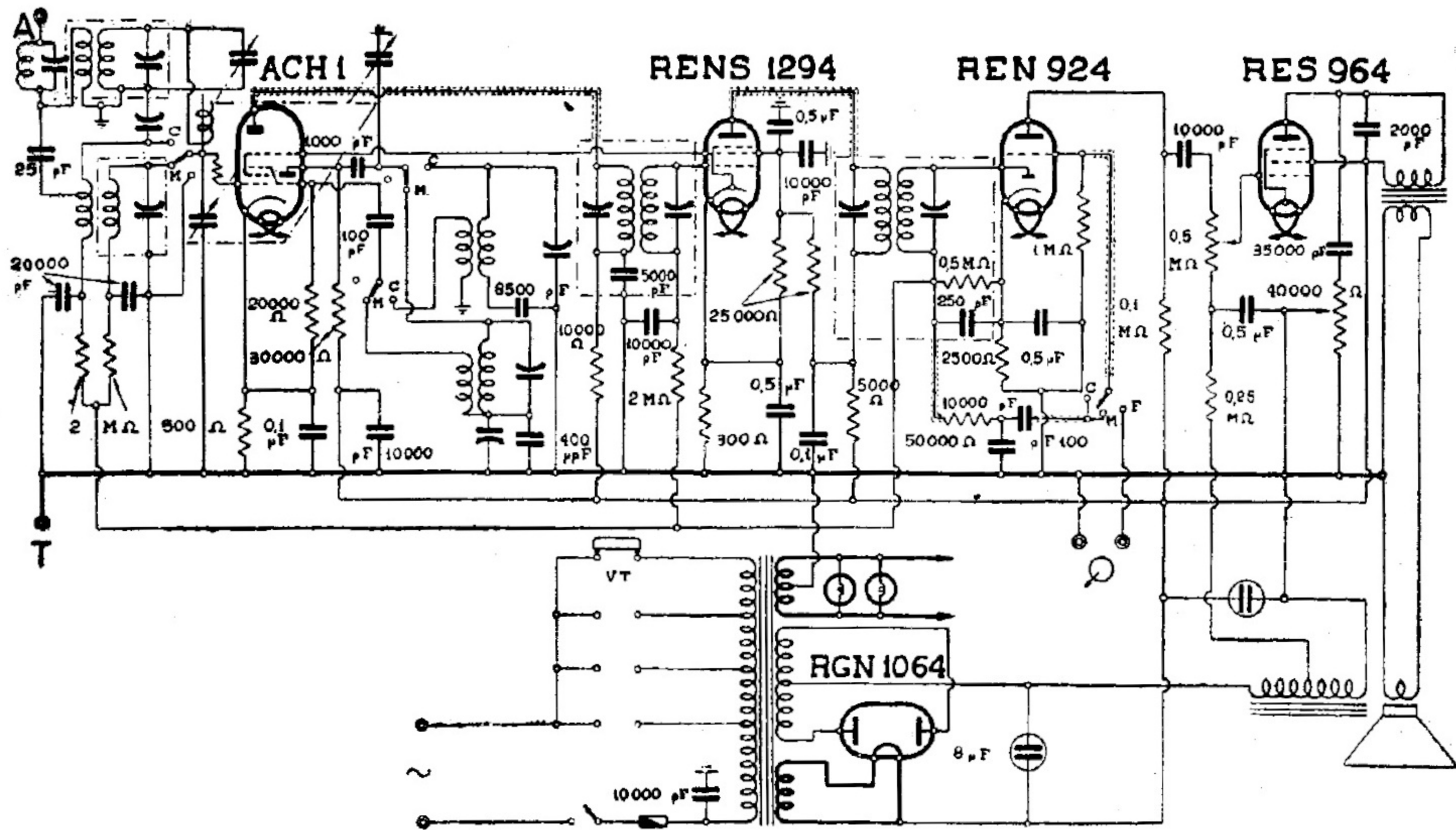
SIEMENS S. A. - MOD. « T 545 »
