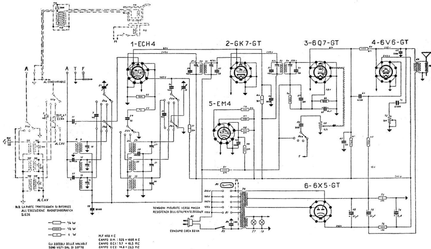
SIEMENS RADIO - Mod. 631 e 636 - Medie e due corte. Media frequenza a 469 kc. Massima tensione raddrizzata 250 V.
