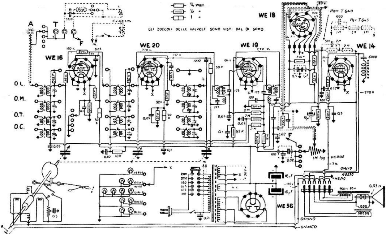
TELEFUNKEN RADIO (S. A. Siemens). — Modello 640 e 645. — Produzione 1939-1940. — Media frequenza: 469 kHz.
