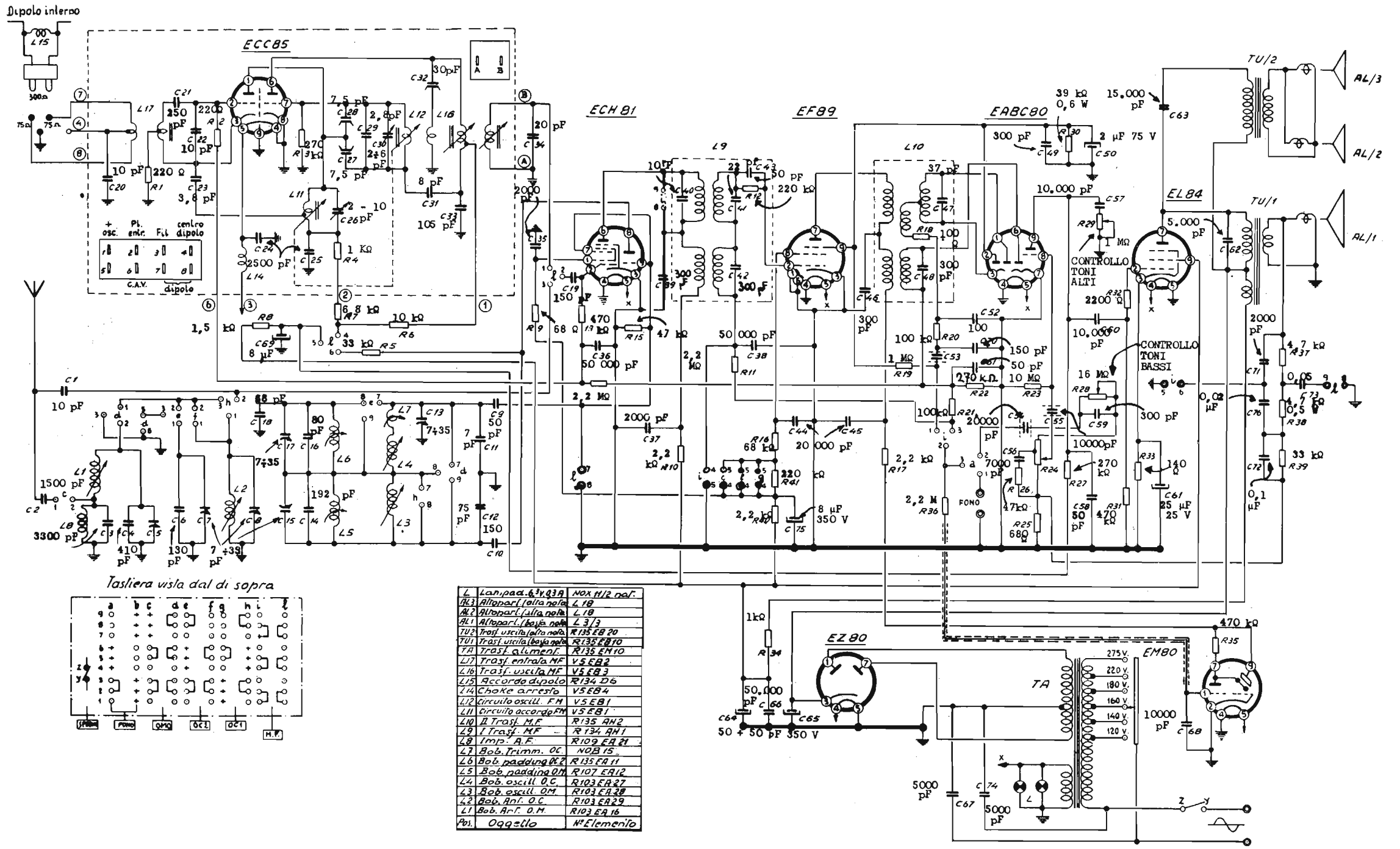
TELEFUNKEN RADIO TV - Mod. MAJESTIC. Apparecchio a modulazione di ampiezza e di frequenza, con suono stereofonico 3D. Onde medie, onde corte, onde cortissime e onde ultracorte (FM). Commutazione d'onda a tastiera. Media frequenza AM a 468 kc/s, media frequenza FM a 10,7 Mc/s. Regolazione dei toni alti e bassi con indicazione visiva. Tre altoparlanti. Potenza d'uscita 4 watt indistorti. (Produzione 1955-56).
