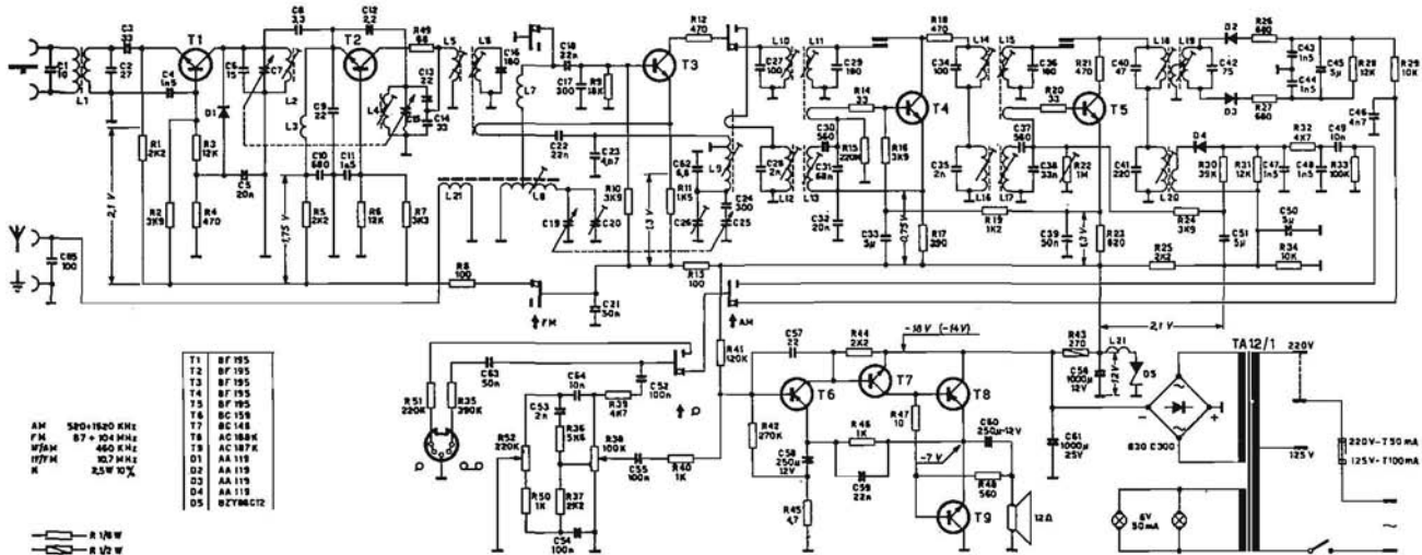
Fig. 3.25. - Schema elettrico di ricevitore AM/FM - (Siemens Eletra mod. RFT662).
