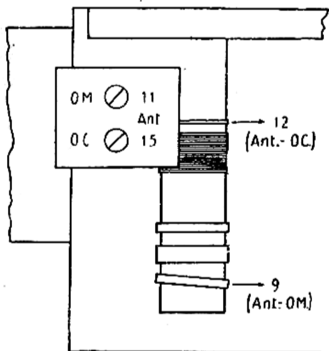
SM 5022 (ANIE) - Posizione dei compensatori.
