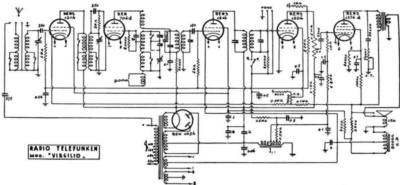
Onde medie e lunghe. - M. F. 175 kc. - C. A. V. - C. T. - Rens 1214 amplif. a. f.; Ren 704d oscill.-modul.; Rens 1214 amplif. m. f.; Rens 1204 demodulatrice-c.a.v.; Rens 1374d finale di potenza. - Potenza d'uscita: 3 watt.
