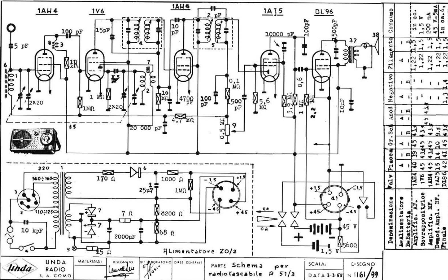
UNDA RADIO - Mod. R 51/3 Mascotte. Apparecchio tascabile, di dimensioni 17×9×4,4 cm. Onde medie da 187 a 570 metri. Quattro valvole subminiatura e una miniatura. Media frequenza a 467 kc/s. Potenza d'uscita 50 mW.
