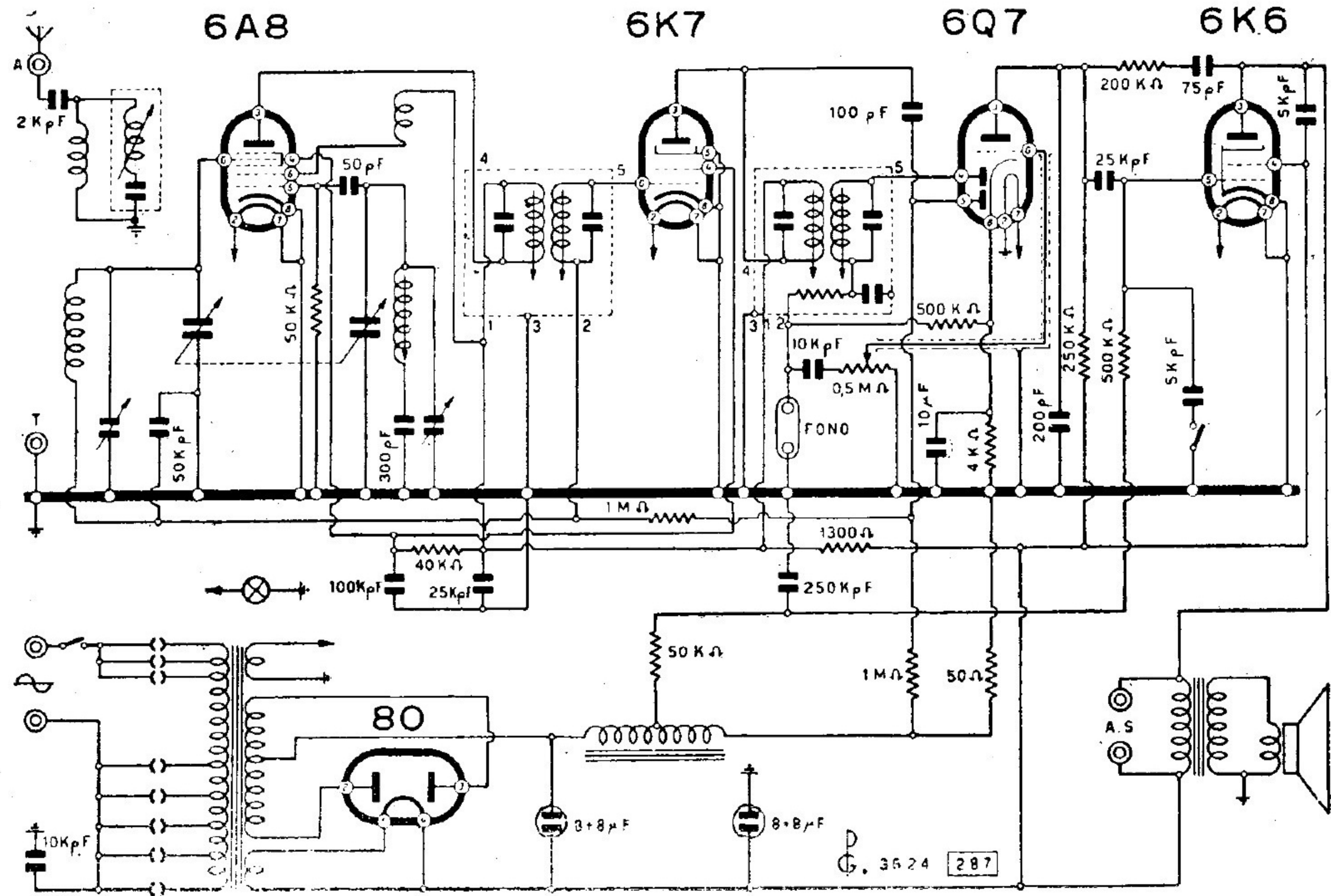
UNDA RADIO - MOD. « MONO UNDA 511 »
