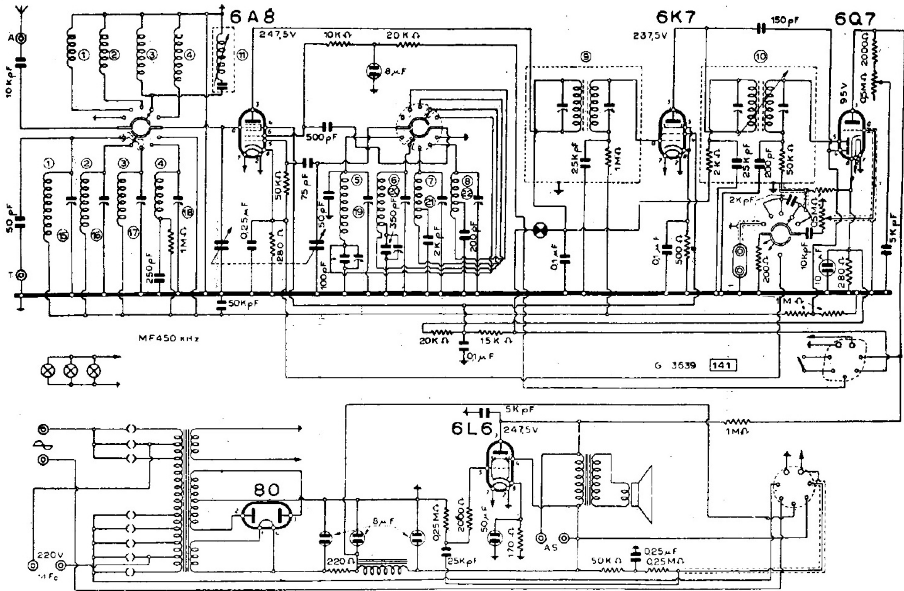
UNDA RADIO - MOD. « QUADRI UNDA 539 »
