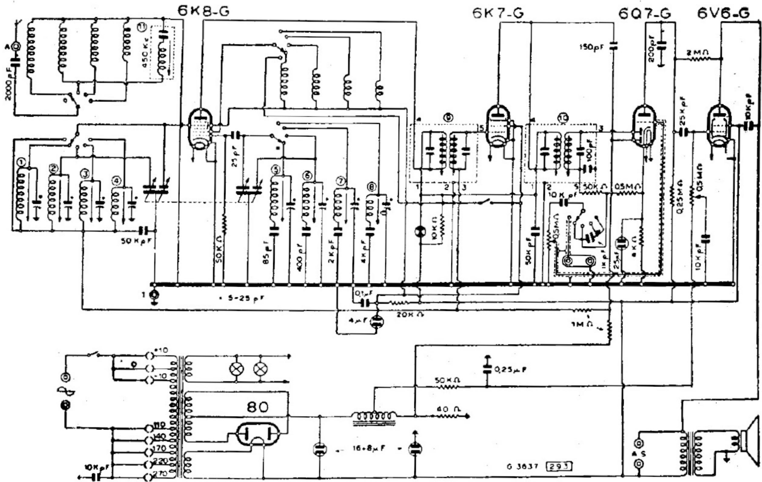
UNDA RADIO - MODD. « QUADRI UNDA 541 » « 543 »
