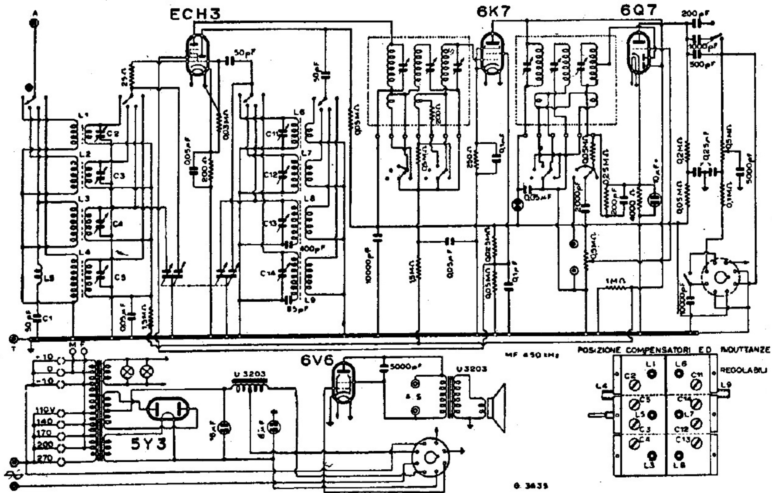
UNDA RADIO - MOD. « QUADRI UNDA 545 »
