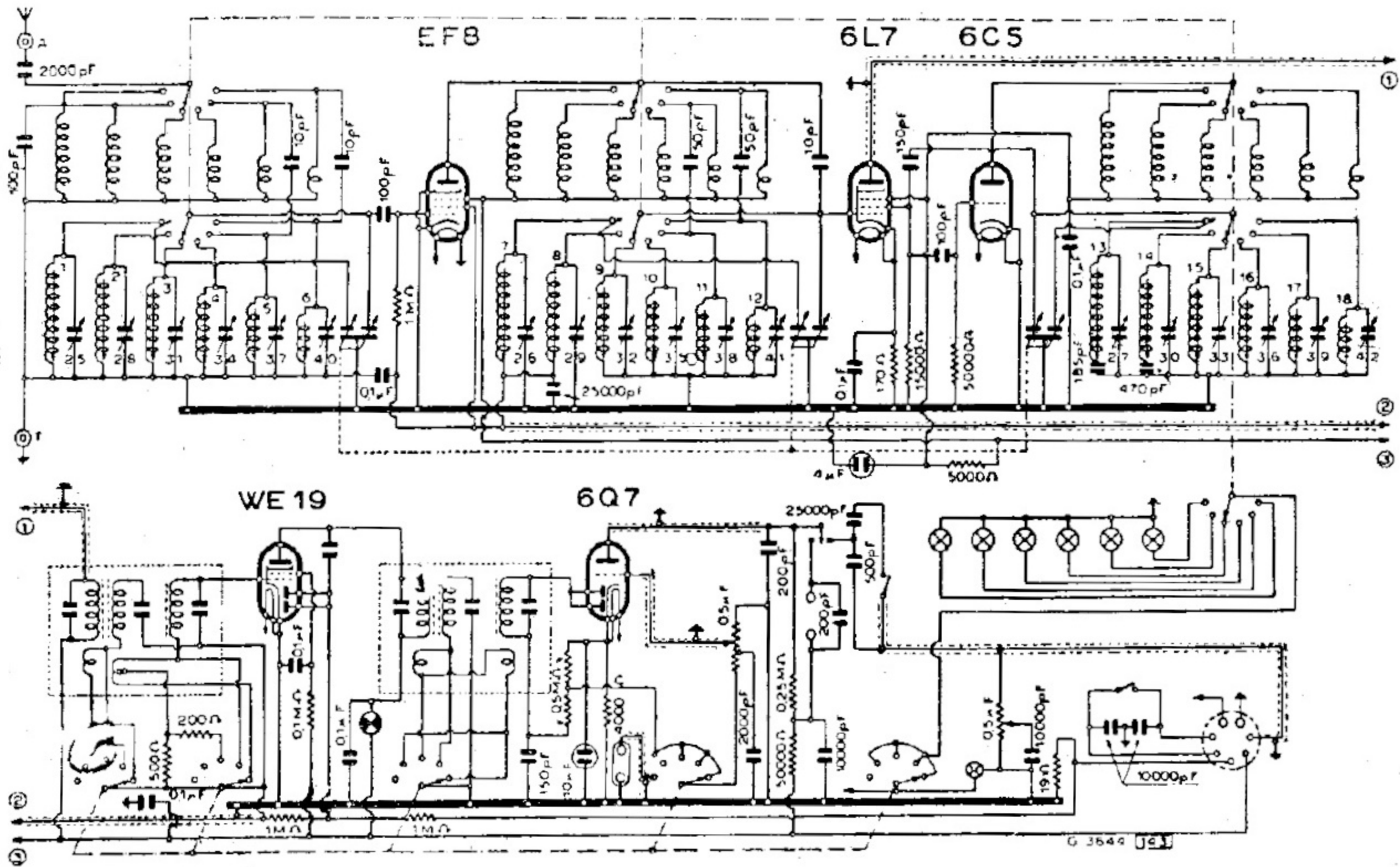
UNDA RADIO - MODD. « SEX UNDA 763 » « 764 »
