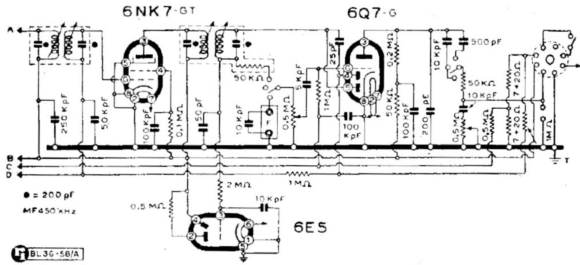
UNDA RADIO - MODD. « OCTA UNDA 78/1 » « 98/1 » PARTE AF - MF
