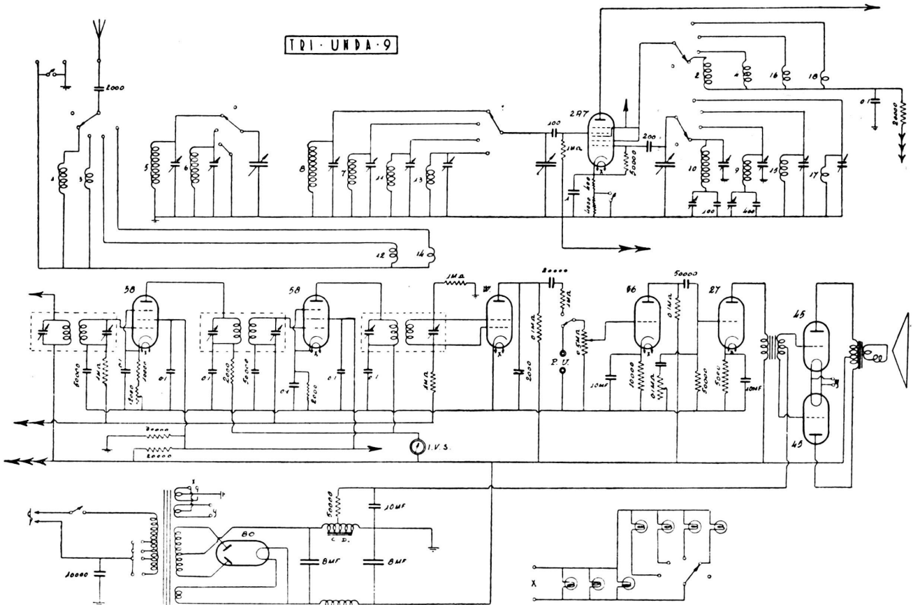
Onde medie, corte e lunghe - M. F. 560 kc. - C. A. V. - C. T. - Scala parlante. - Controfase di 15. - Potenza d'uscita: 9 watt.
