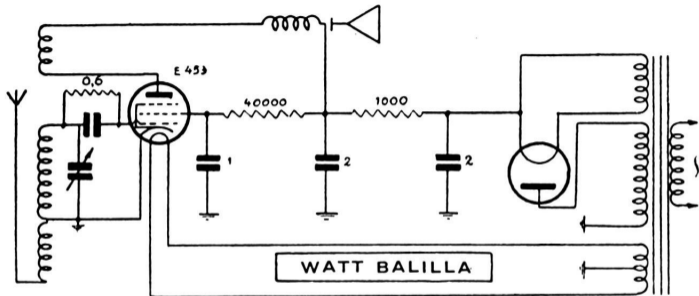
Valvola schermata in reazione, per la ricezione della emittente locale, alimentata con una rettificatrice monoplacca.
