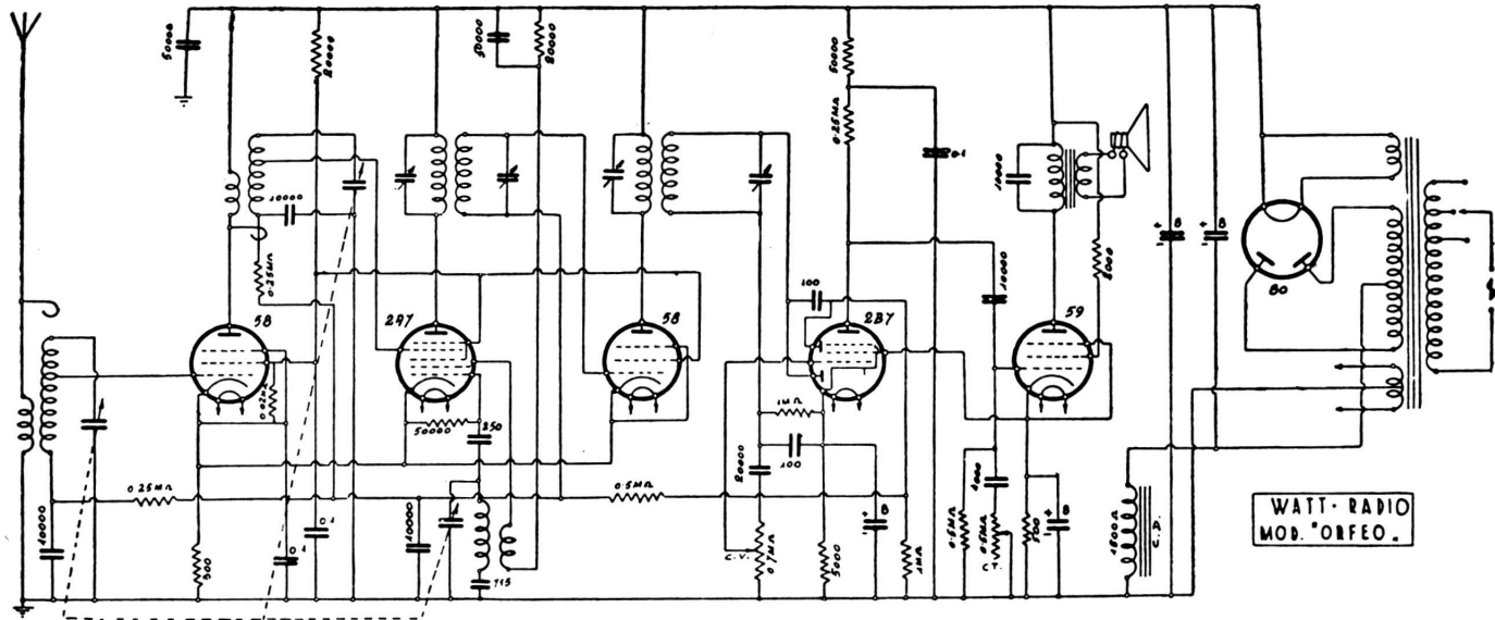
Onde medie. - M. F. 175 kc. - C. A. V. - C. T. - 58 amplif. a. f. (pl. 260 v., sch. 90 v.), 2A7 oscill.-modul. (pl. 260 v., sch. 90 v.), 58 amplif. m. f. (pl. 260, sch. 90), 2B7 demod.-c.a.v. (pl. 200 v. sch. 18 v., gr. 3,1 v.), 59 finale di potenza (pl. 250 v., sch. 250 v., gr. 18 v.). - Potenza d'uscita: 3,5 watt.
