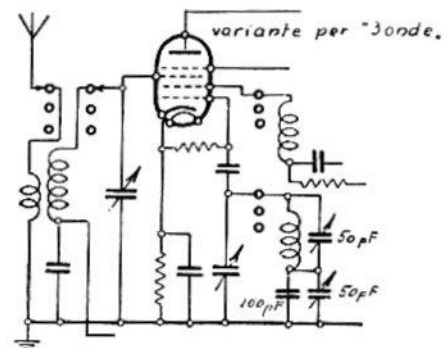
WATT RADIO. — Mod. « Super Stella » e « Super Stella Fono ». — Produzione 1940-1941. Media frequenza: 460 kHz.
